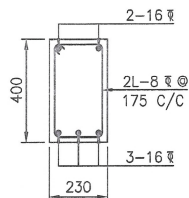
SECTION T-T (SCALE 1:20)
