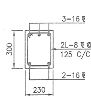
SECTION V-V (SCALE 1:20)
