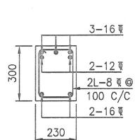
SECTION S-S (SCALE 1:20)
